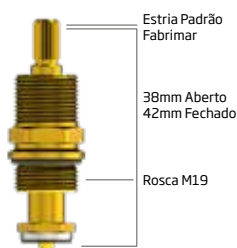
1416 MVS Cód. 26603 1416 Fabrimar
