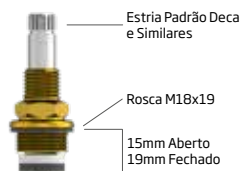
TORNEIRA SV Cód. 6582 Linha Stander / Universal
