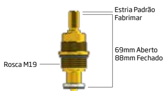
TORNEIRA MVS Cód. 15437 Fabrimar
