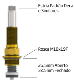
1416 1/2 e 3/4 SV Cód. 21954 Linha 1416 1/2 e 3/4 Real e Similares
