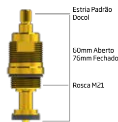
1416 MVS Cód. 10004 1416 Docol
