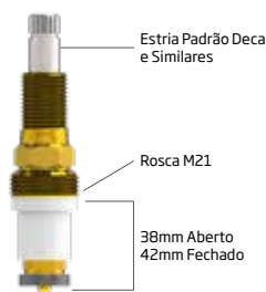
1416 MVS Longo Cód. 6573 Linha Universal
