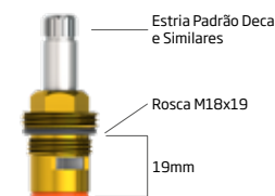
1/4 DE VOLTA M18 Cód. 15686 Linha Stander / Universal
